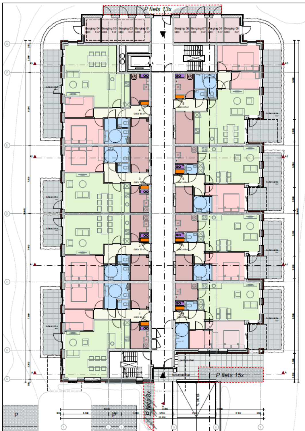
Figuur 33: Plattegrond begane grond met fietsparkeerplaatsen voorzien van een rode omlijn
